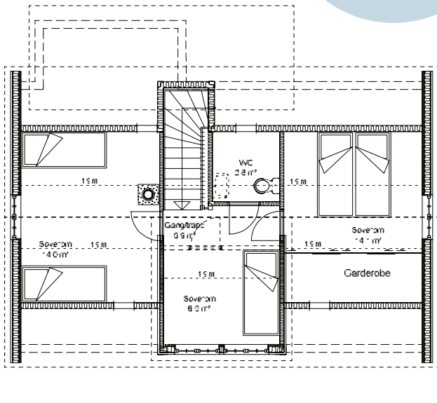
Hems: Gang, tre soverom, WC og terrasse
