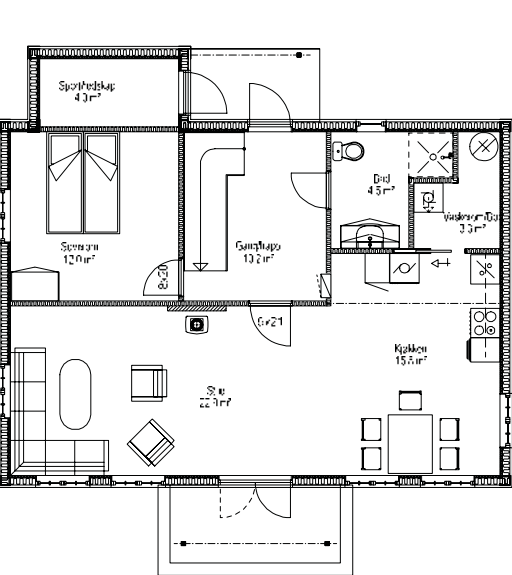
Grunnplan: Stue, kjøkken, soverom, bad,vask/bod og sportsbod
