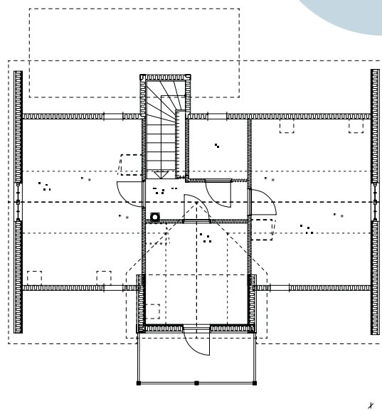
Hems: Gang, tre soverom, WC og terrasse.
